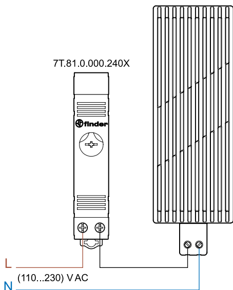
Схема подключения AC
