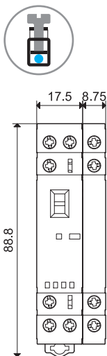
Тип 22.32 + 022.33/022.35 Винтовые клеммы
