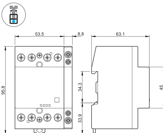
Тип 22.44/22.64 + 022.63/022.65 Винтовые клеммы
