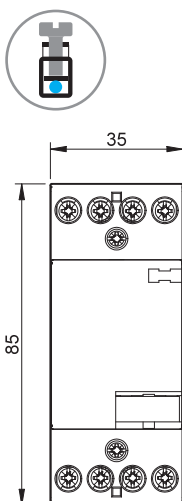
Тип 22.74 Винтовые клеммы
