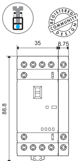
Тип 22.34 + 022.33/022.35 Винтовые клеммы
