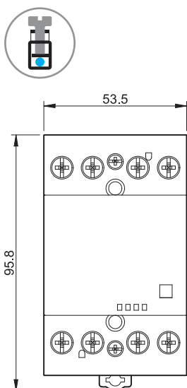
Тип 22.44/22.64 Винтовые клеммы
