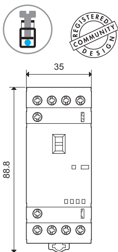
Тип 22.34 Винтовые клеммы
