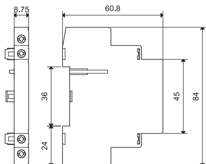
Тип 022.73/022.75 Винтовые клеммы
