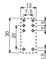
95.15.2 Вид сбоку
