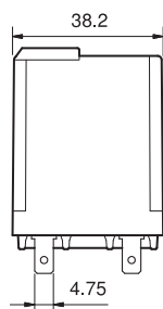
Тип 62.32 62.32-4300
