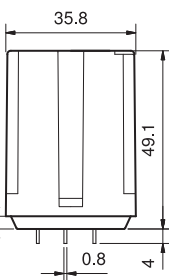
Тип 62.3x-4300
