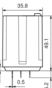
Тип 62.8x-4300
