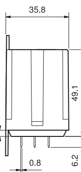
Тип 62.8x-4300
