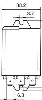
Тип 62.83 62.83-4300
