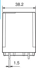
Тип 62.22 62.22-4300
