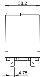
Тип 62.32-4800
