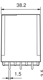
Тип 62.23 62.23-4300
