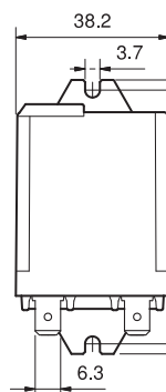
Тип 62.82 62.82-4300
