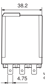
Тип 62.33 62.33-4300
