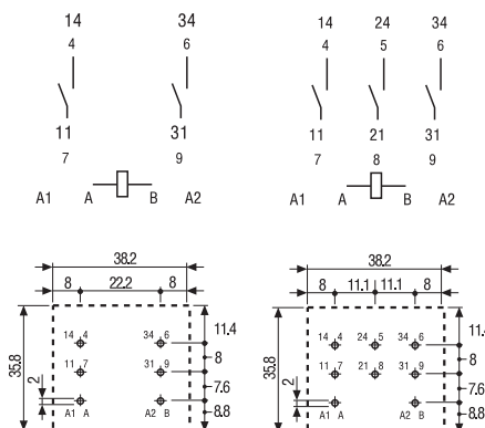
62.22 - 4300 Вид со стороны выводов
