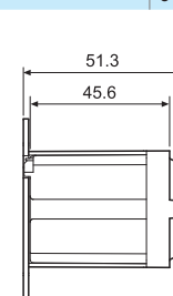
062.05 с реле
