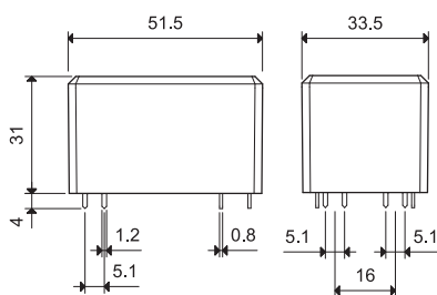
Тип 66.22-х600S
