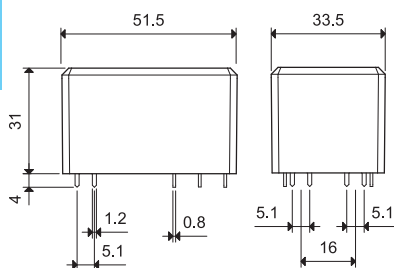
Тип 66.22-х300
