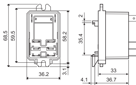
066.07 с реле
