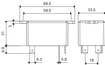
Тип 66.82-х300
