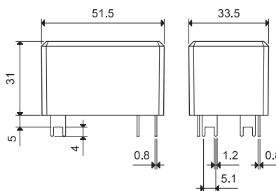
Тип 66.22-х600S
