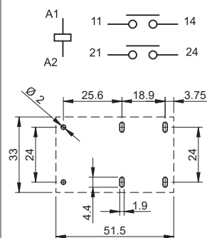
Вид со стороны выводов
