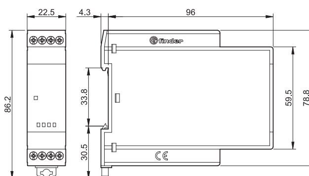
Тип 7S.36 Винтовые клеммы
